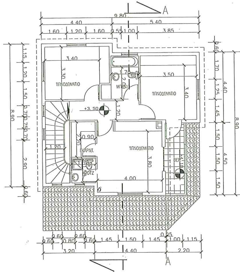
ΚΑΤΟΨΗ ΟΡΟΦΟΥ
