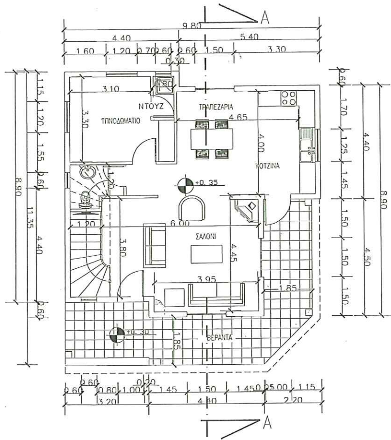
ΚΑΤΟΨΗ ΙΣΟΓΕΙΟΥ
